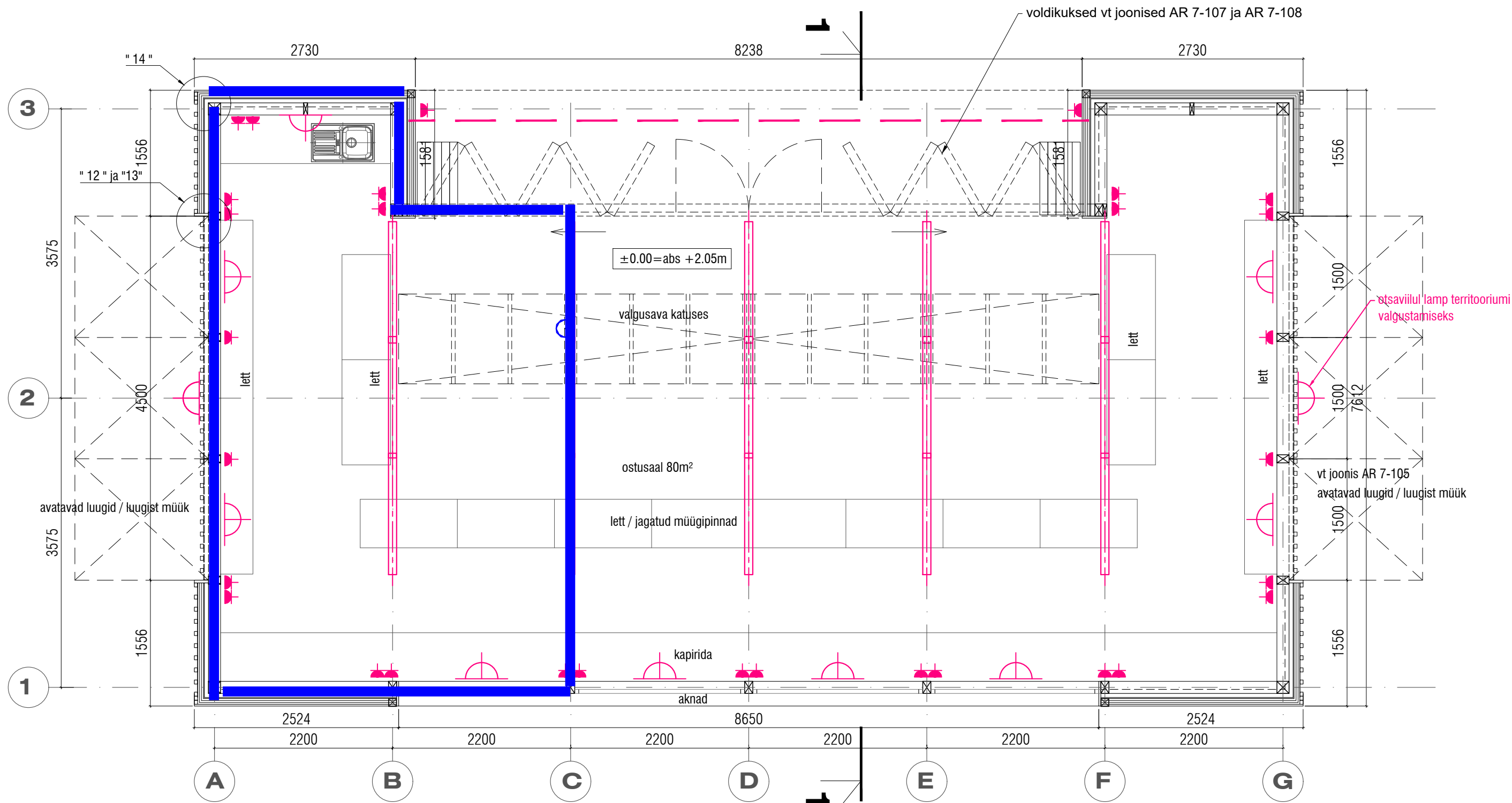
1 PÕHIPLAAN M 1:50
